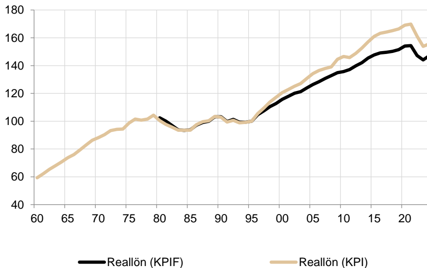
Diagram 1. Reallön i nivå sedan 1960. Index, 1995 = 100
